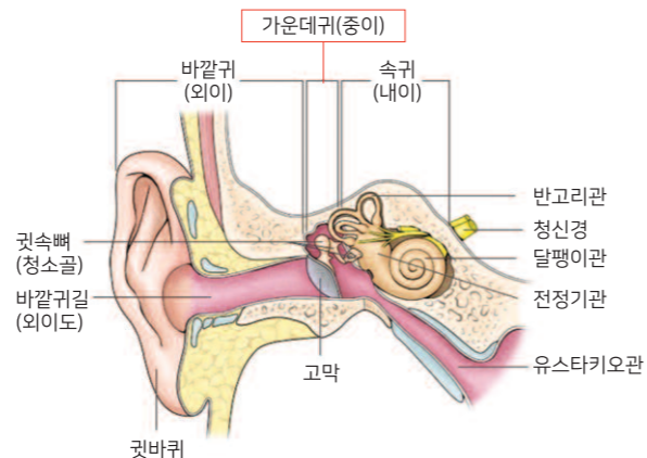
그림 1. 귀의 구조
